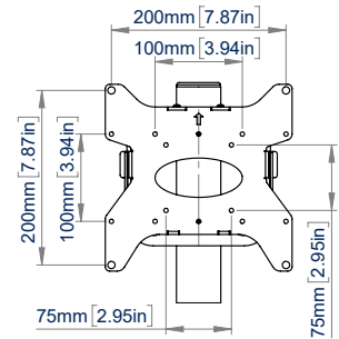
SCALE 1 : 6
