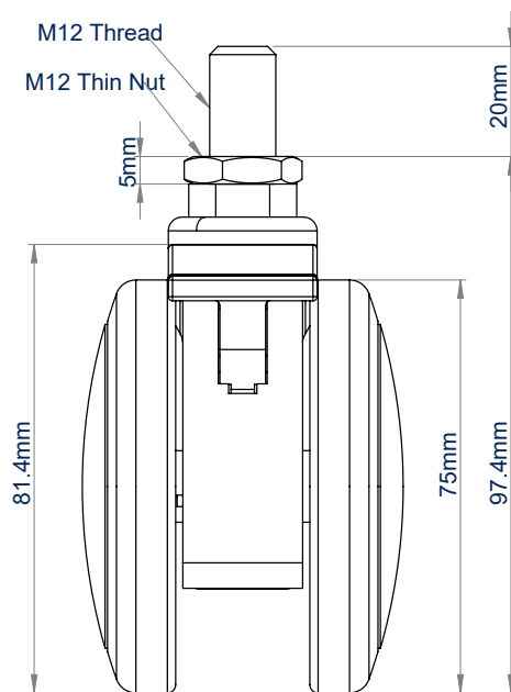
VOORAANZICHT
