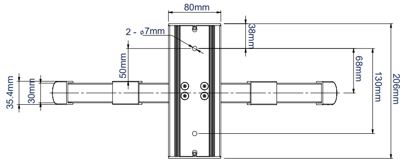
ACHTERAANZICHT
