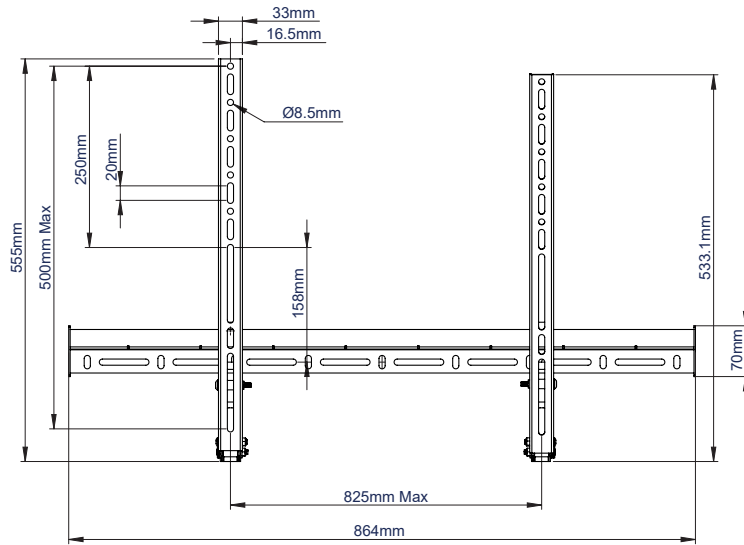
VOORAANZICHT
