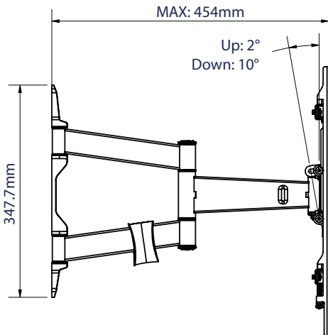
ZIJAANZICHT MAXIMALE UITREKking
