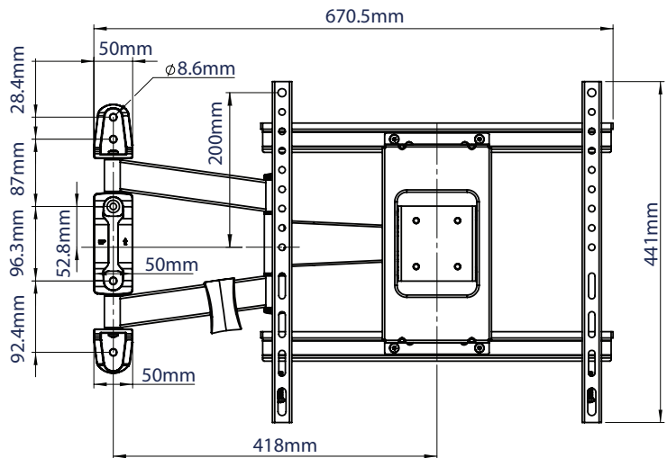
VOORAANZICHT MET DE ARM NAAR DE ZIJKANT UITGESTREKT
