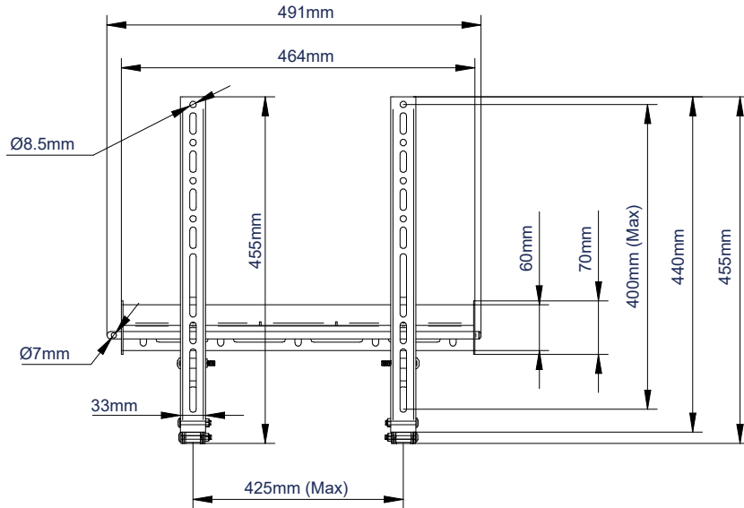
VOORAANZICHT
