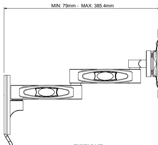
ZIJZICHT ARM GESTREKT
