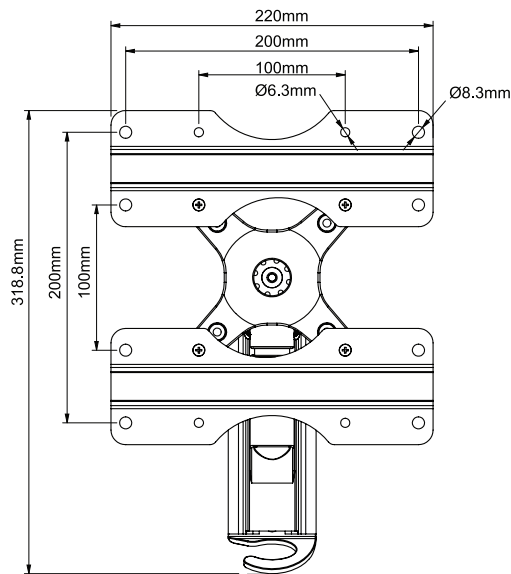
VOORAANZICHT VOLLEDIGE UITSCHUIFLENGTE
