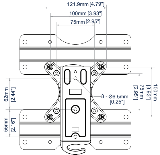
ACHTERKANT
