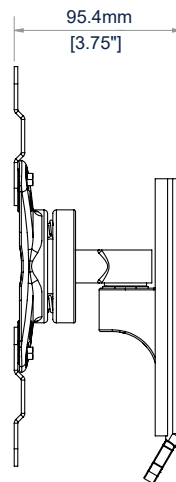
ZIJZICHT
