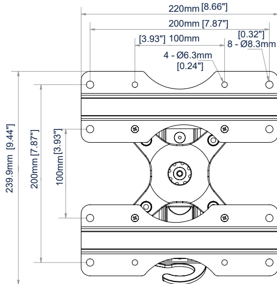
VOORAANZICHT
