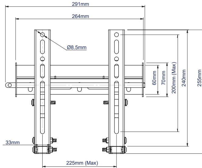
VOORAANZICHT
