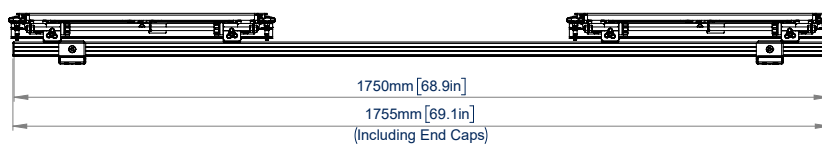
BOVENAANZICHT
