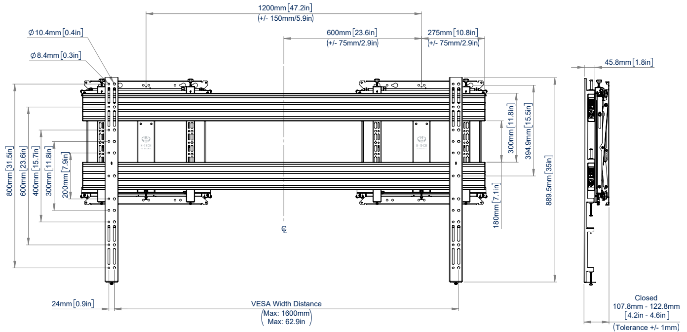
VOORAANZICHT
