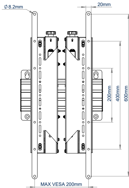
VOORAANZICHT
