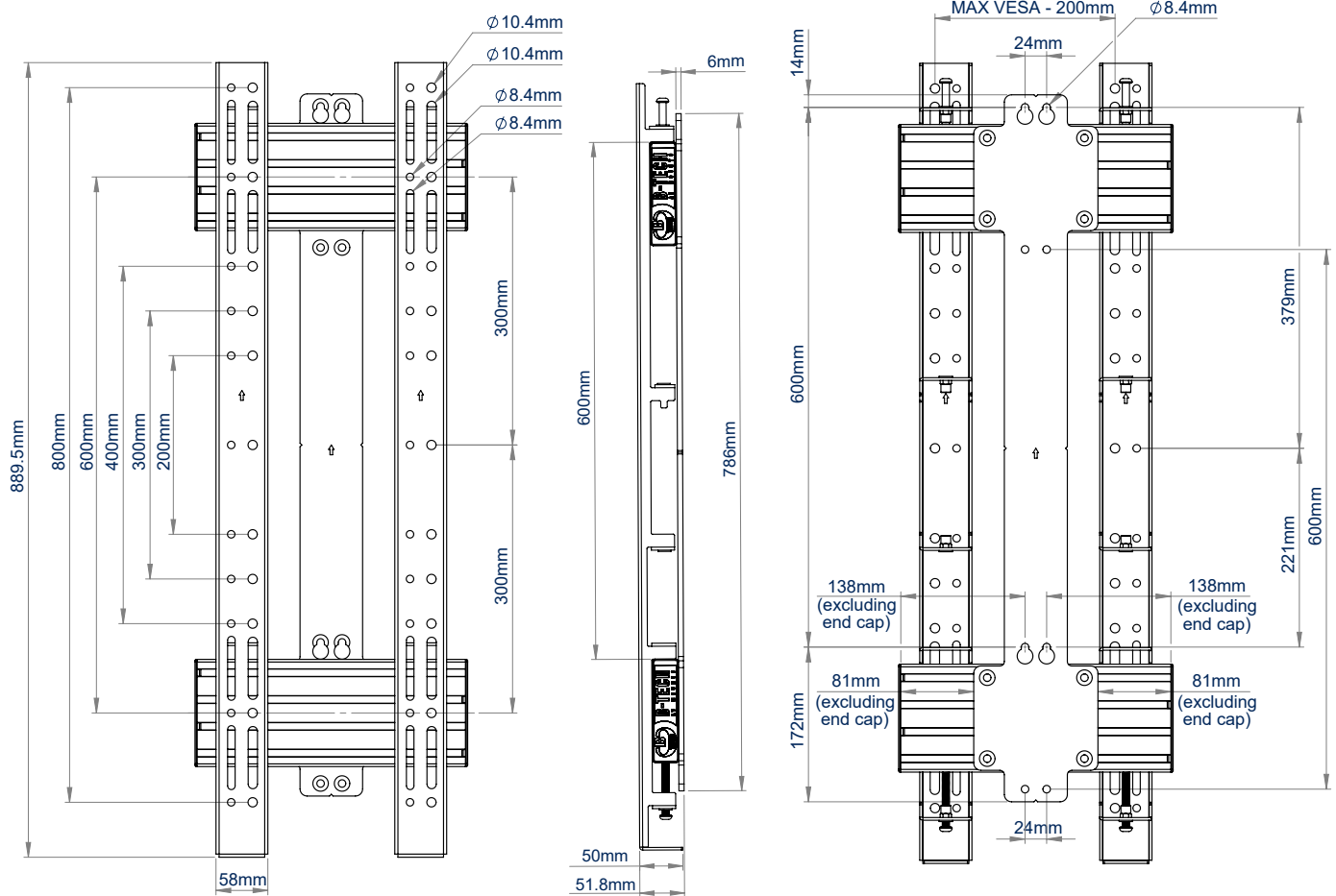
VOORAANZICHT
