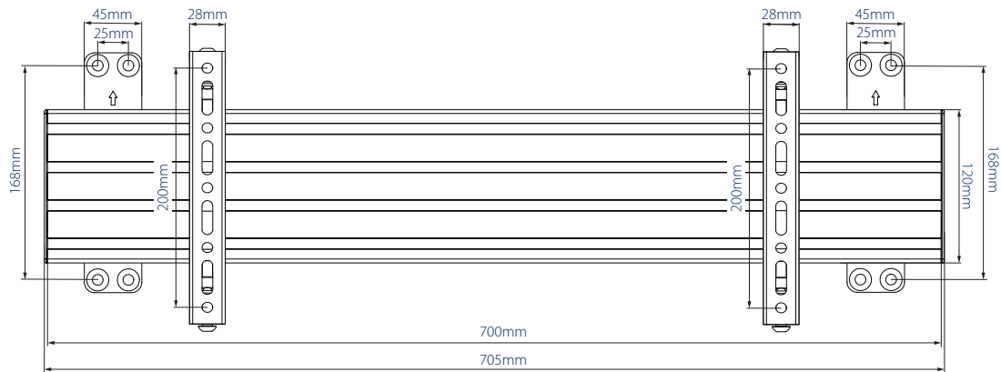
VOORAANZICHT
