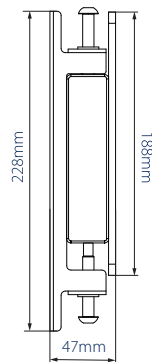
ZIJAANZICHT
