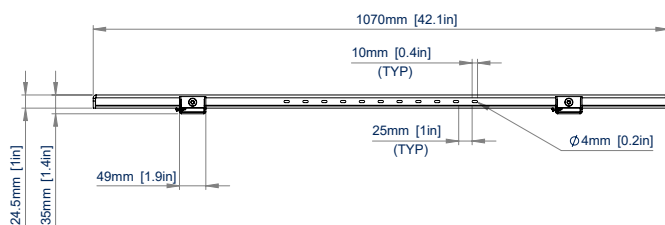
BOVENAANZICHT
