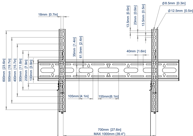
VOORAANZICHT
