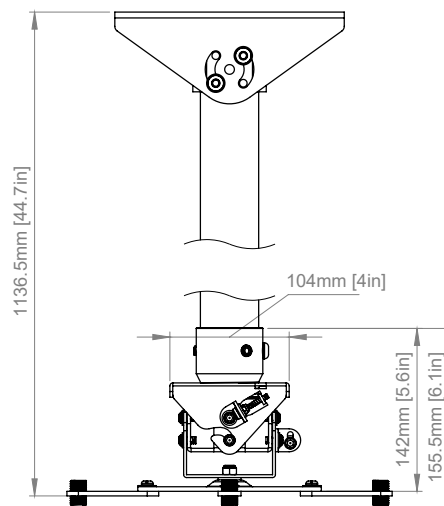
ZIJAANZICHT
