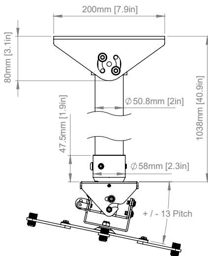
ZIJAANZICHT
