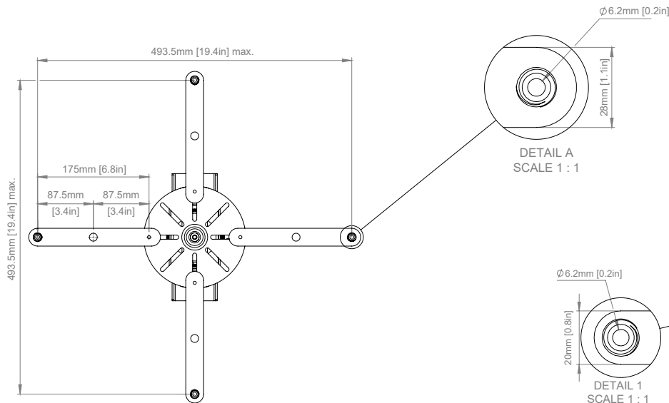
AANZICHT VAN ONDERAF
