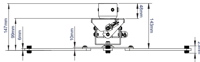
ZIJAAANZICHT / PLAT MET GEMONTEERDE STANGADAPTER
