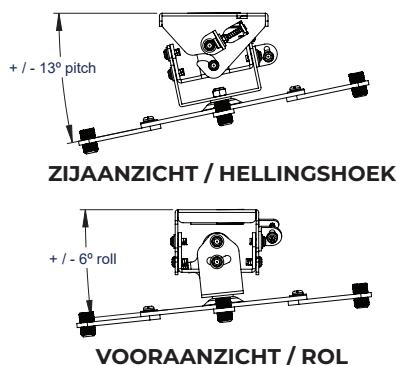
VOORAANZICHT / ROL
