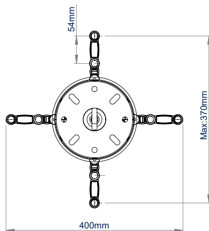
AANZICHT VAN ONDERAF
