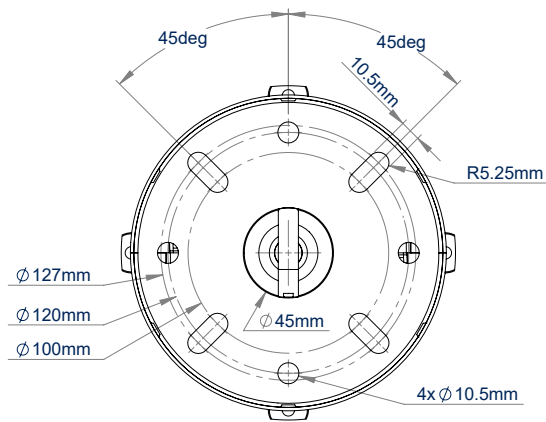
BOVENAANZICHT
