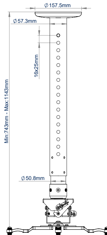
VOORAANZICHT
