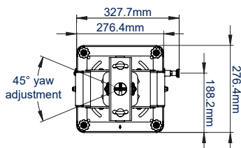
BOVENAANZICHT
