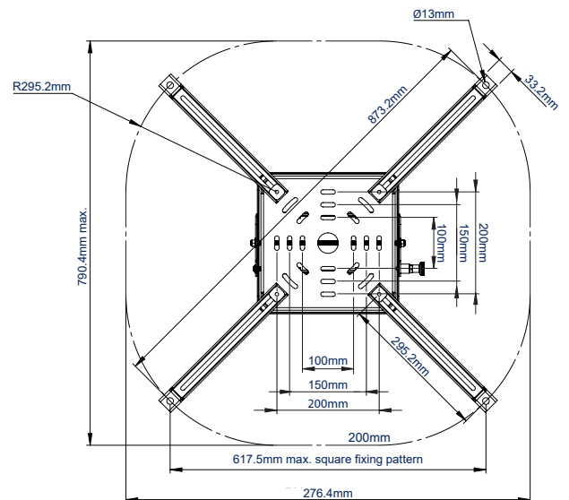
AANZICHT VAN ONDERAF MET LANGE UITSCHUIFBARE POTEN
