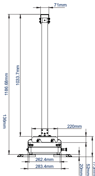
VOORAANZICHT MET UITSCHUIFBARE POTEN
