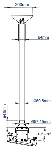
ZIJAANZICHT KANTELING WEERGEVEN
