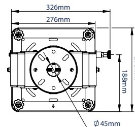
BOVENAANZICHT MET PLAFONDPLAAT
