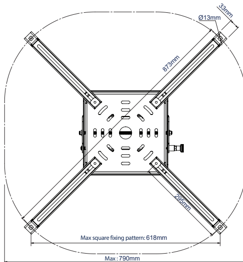
INTERFACE MET LANGE UITSCHUIFBARE POTEN & KORTE UITSCHUIFBARE POTEN
