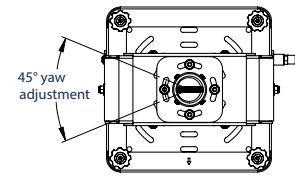
BOVENAANZICHT
