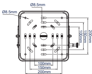
AANZICHT VAN ONDERAF AANSLUITPLAAT
