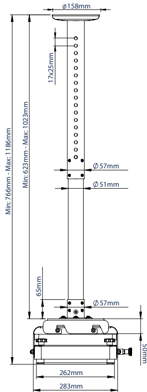
VOORAANZICHT
