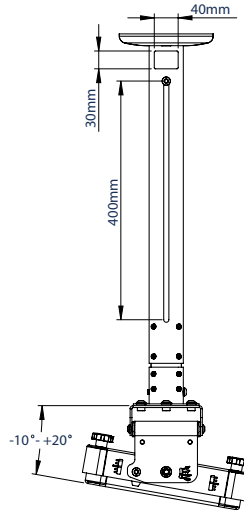
ZIJZICHT MET INTERFACE TILT
