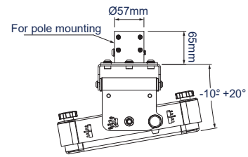
ZIJAANZICHT INCLUSIEF STANGADAPTER
