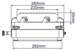
VOORAANZICHT
