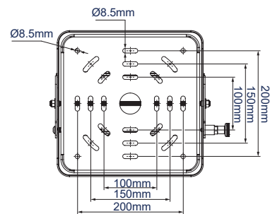
AANZICHT VAN ONDERAF
