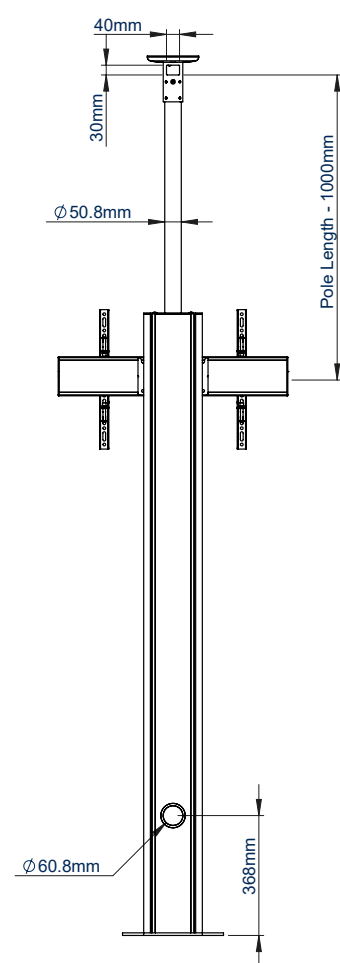
ACHTERAANZICHT
