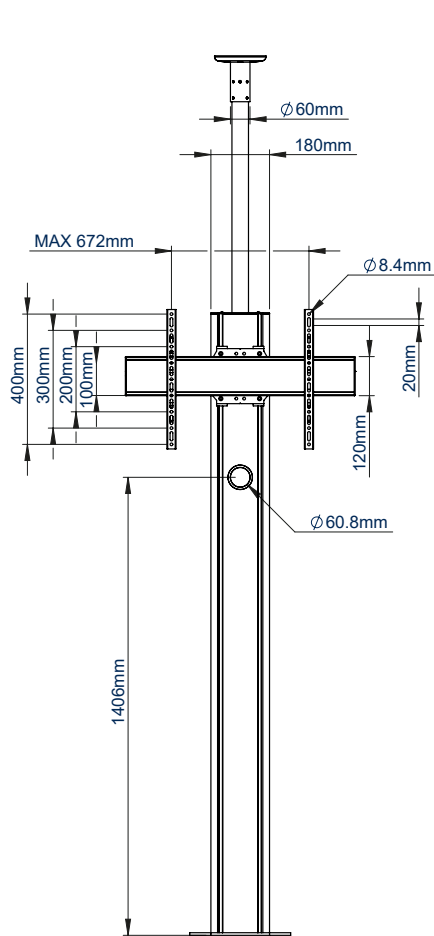
VOORAANZICHT
