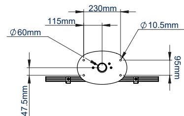
ACHTERAANZICHT
