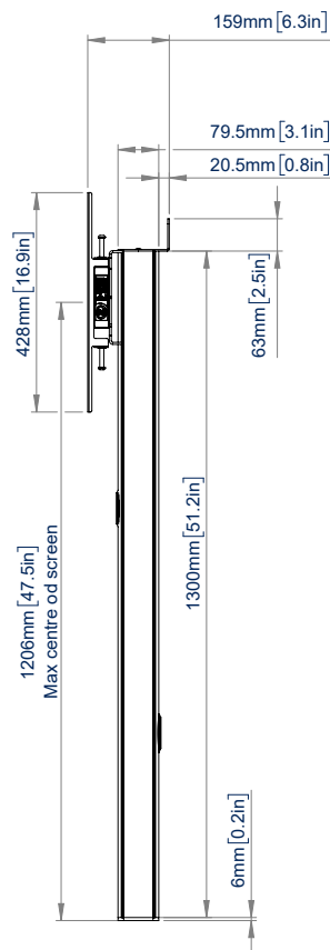
ZIJZICHT
