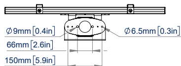
BOVENAANZICHT
