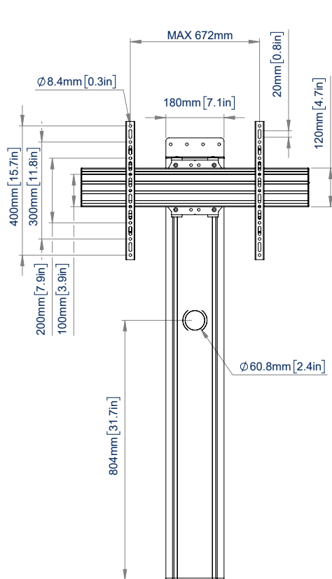
VOORAANZICHT
