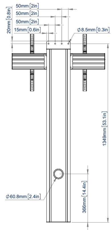
ACHTERAANZICHT
