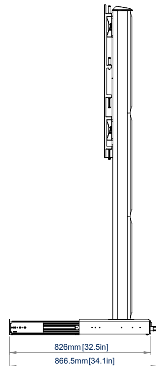
ZIJAANZICHT UITGEBREID
