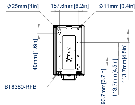
AANZICHT VAN ONDERAF INTREKBARE VOET
