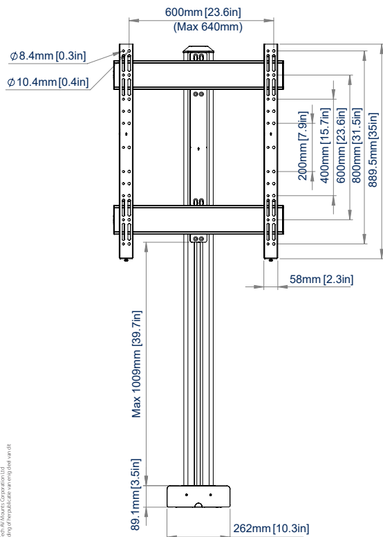
VOORAANZICHT
