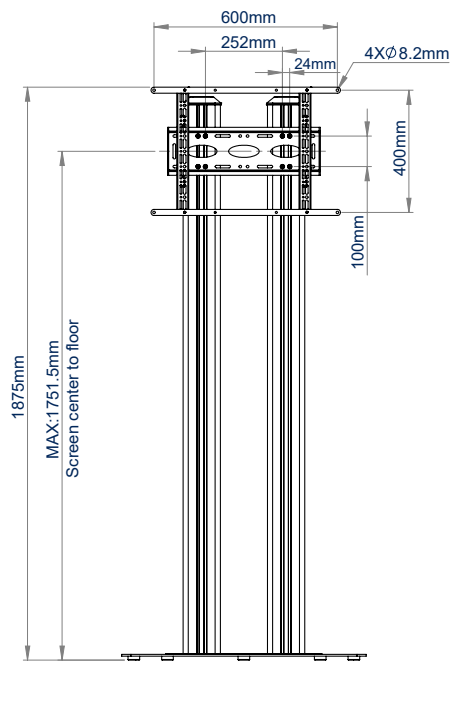
VOORAANZICHT
