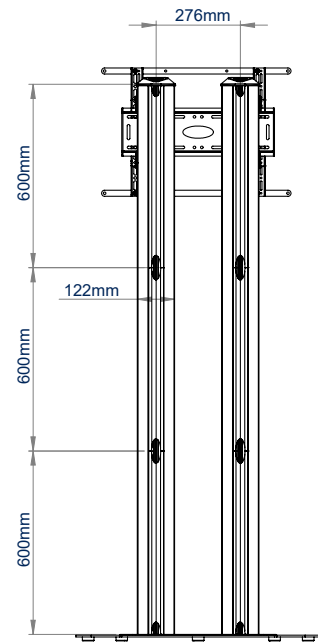
ACHTERAANZICHT
