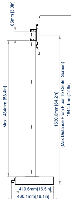
ZIJAANZICHT
