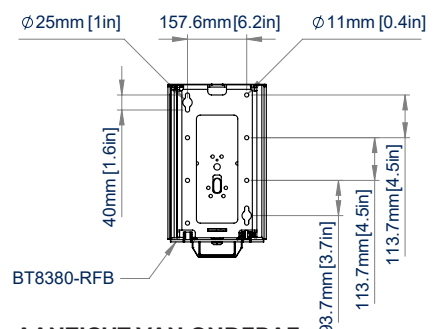
AANZICHT VAN ONDERAF INTREKBARE VOET
