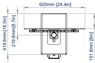
BOVENAANZICHT
