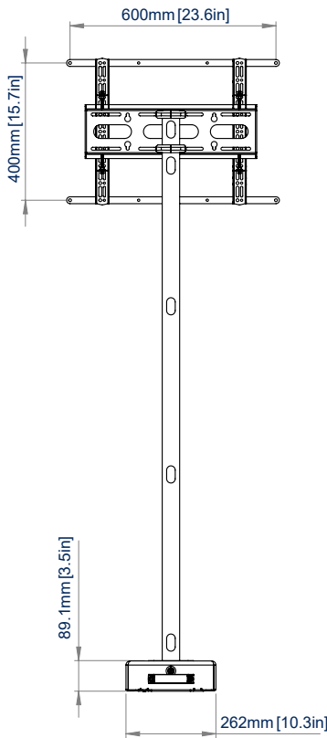
ACHTERKANT
