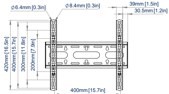
VOORAANZICHT INTERFACE
