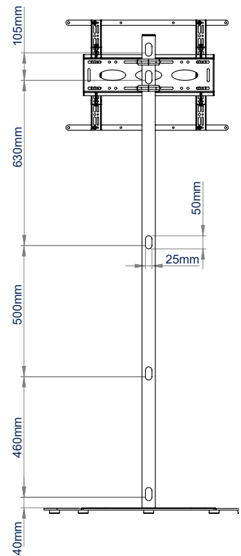
ACHTERAANZICHT
