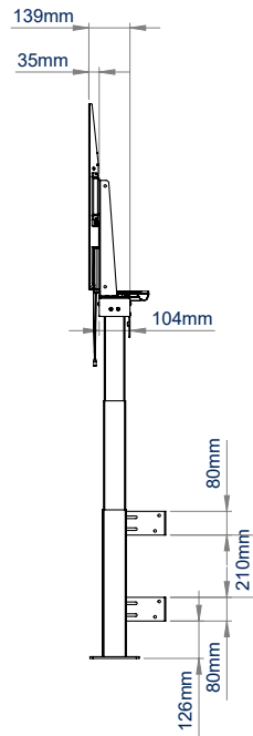
ZIJAAANZICHT
