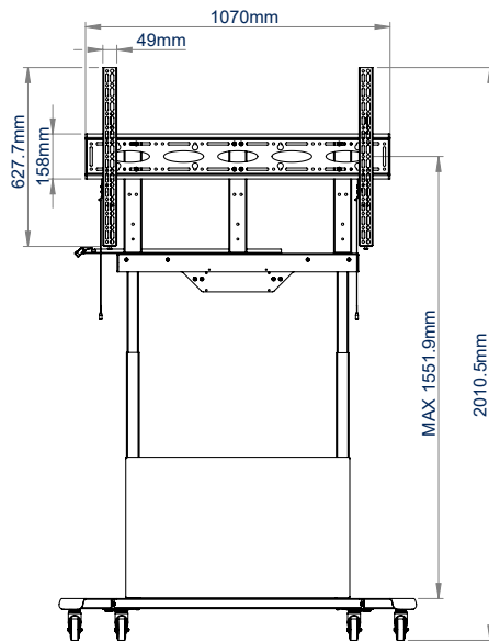
VOORAANZICHT HOOGSTE FUNCTIE
