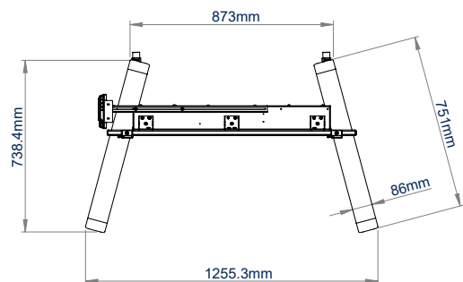
BOVENAANZICHT
