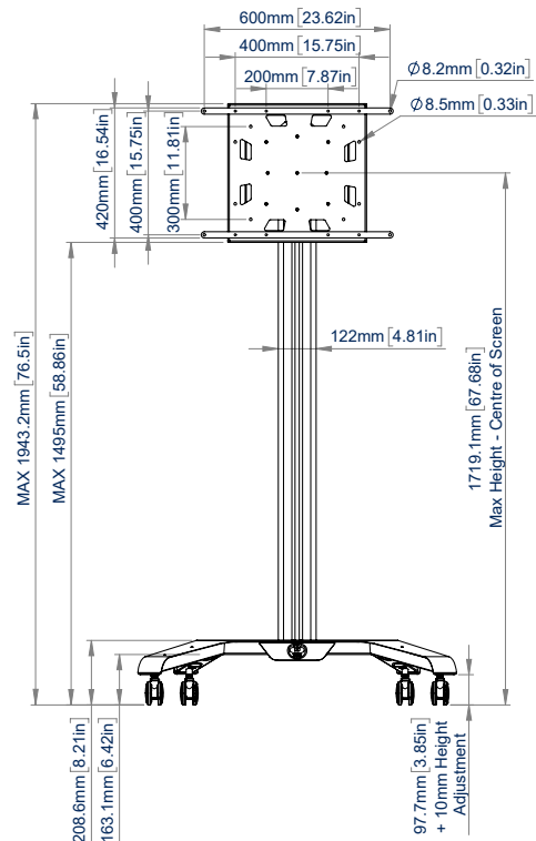
VOORAANZICHT
