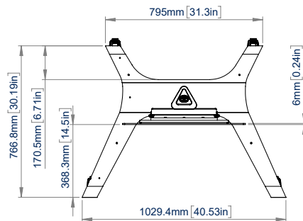
BOVENAANZICHT
