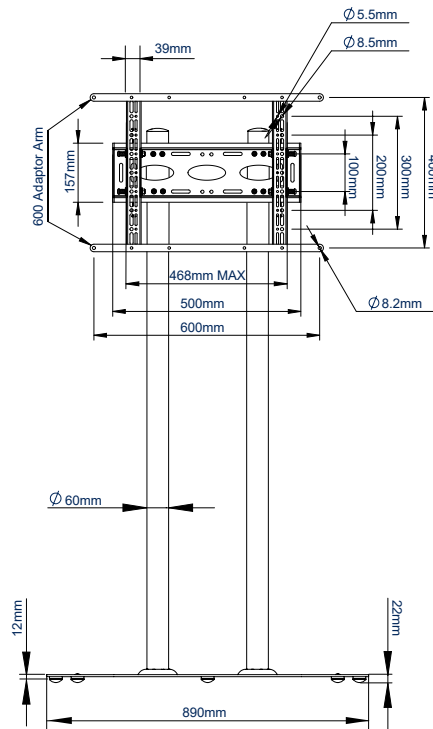
VOORAANZICHT
