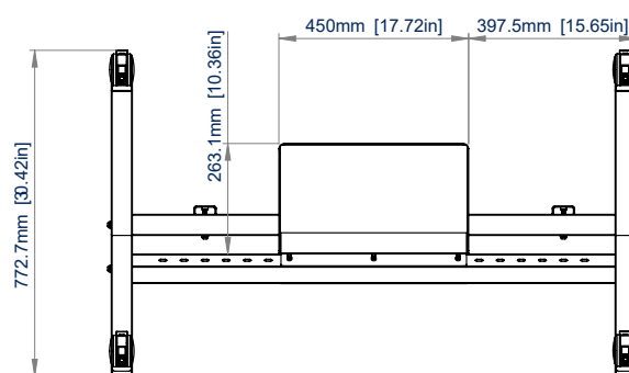
BOVENAANZICHT
