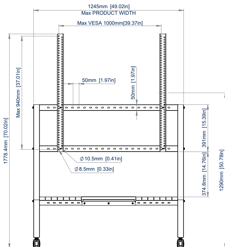
VOORAANZICHT
