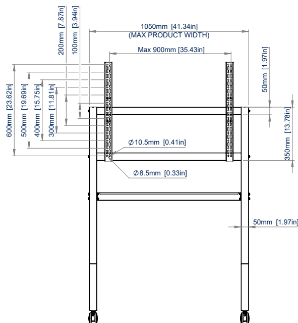
VOORAANZICHT
