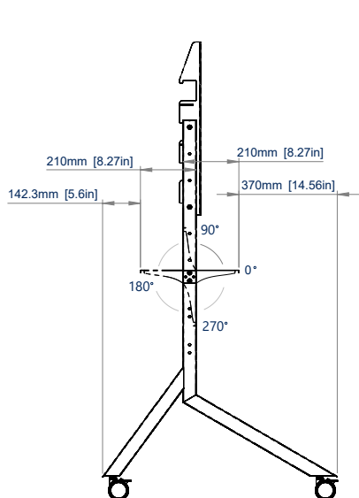
AANZICHT VAN DE RECHTERZIJDE MINIMALE LENGTE
