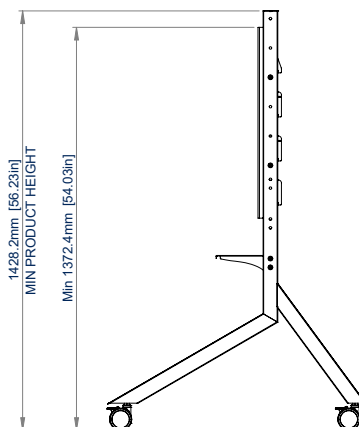
AANZICHT VANAF DE LINKERKANT MINIMALE LENGTE
