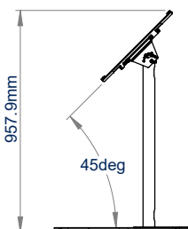
45° KANTELING
