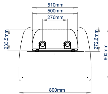
STANDAARD BASE
