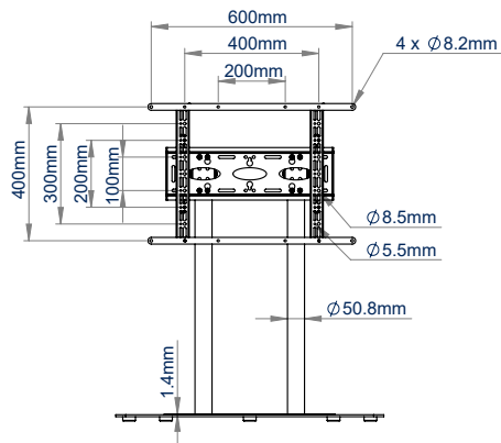
VOORAANZICHT
