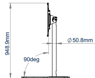
90° KANTELING
