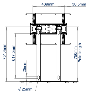
ACHTERAANZICHT
