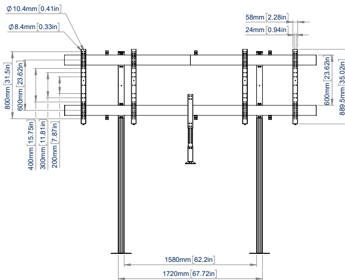
VOORAANZICHT
