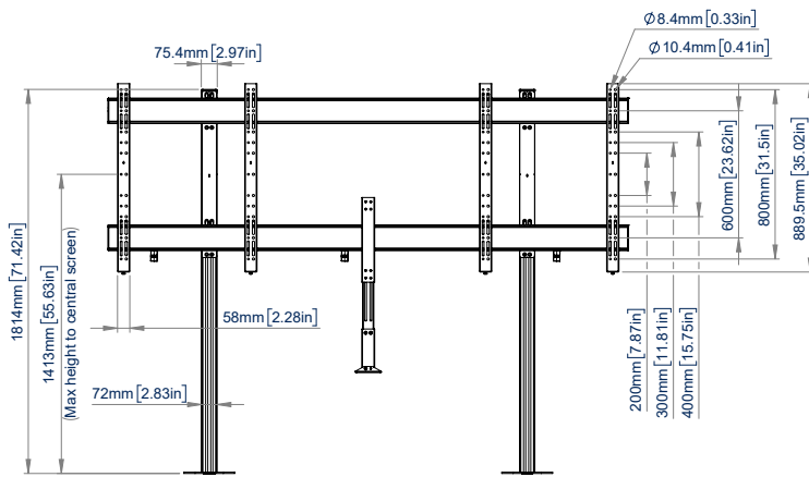
VOORAANZICHT
