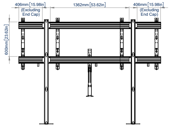
ACHTERKANT
