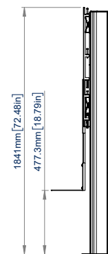
ZIJZICHT
