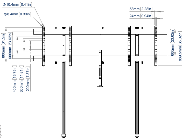
VOORAANZICHT
