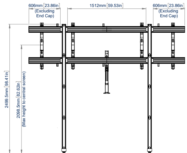
ACHTERAANZICHT
