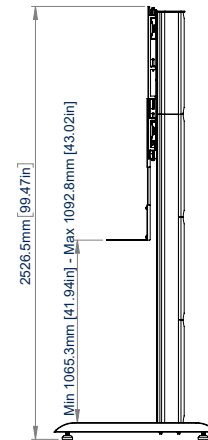
ZIJAANZICHT
