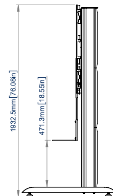
ZIJZICHT
