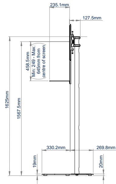
ZIJAANZICHT
