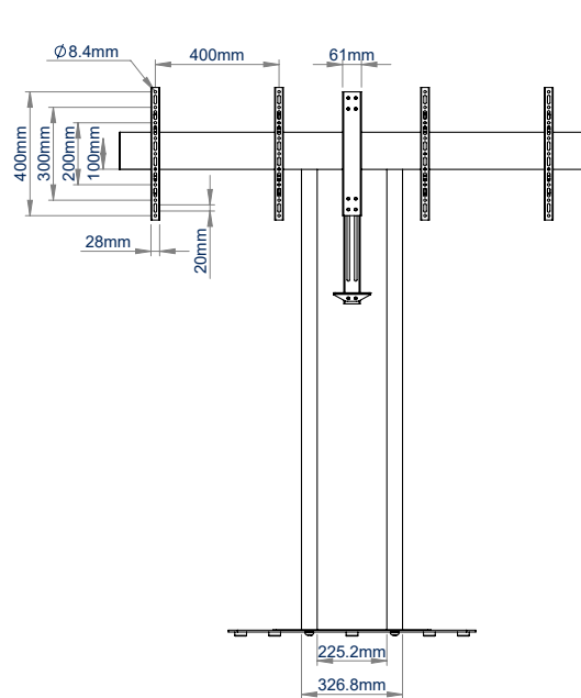
VOORAANZICHT
