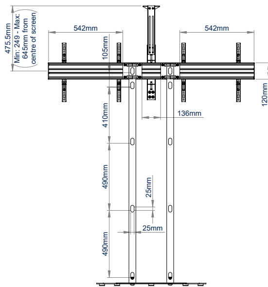
ACHTERAANZICHT
