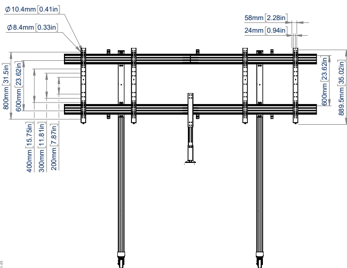
VOORAANZICHT
