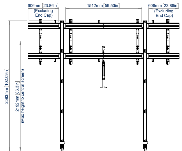
ACHTERAANZICHT
