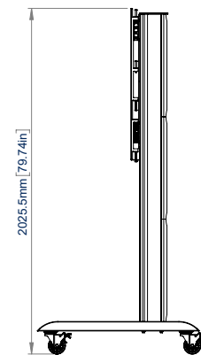
ZIJAANZICHT
