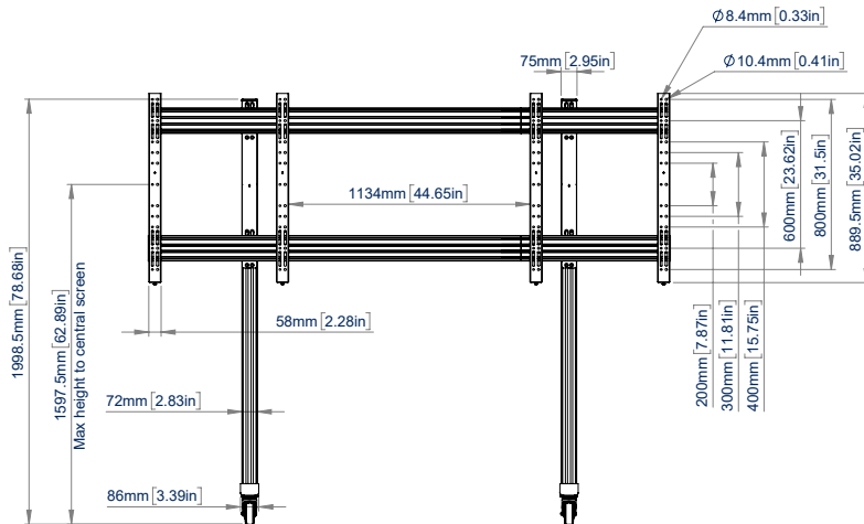
VOORAANZICHT
