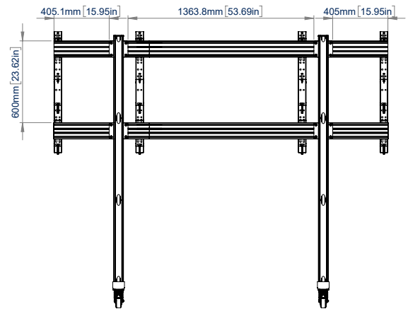
ACHTERAANZICHT
