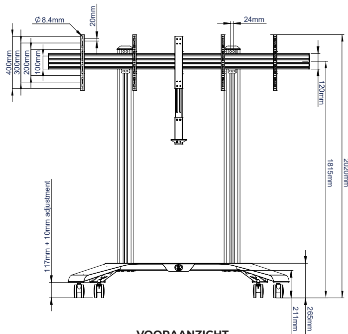
VOORAANZICHT
