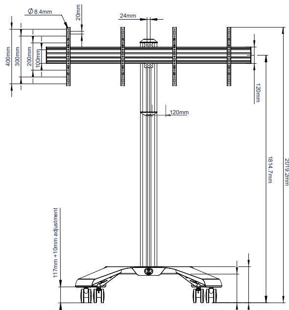
VOORAANZICHT
