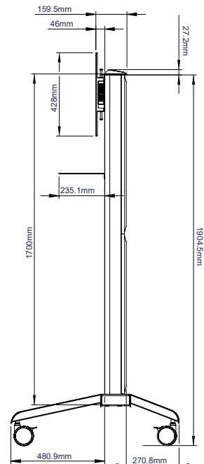
ZIJAANZICHT
