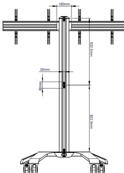
ACHTERAANZICHT
