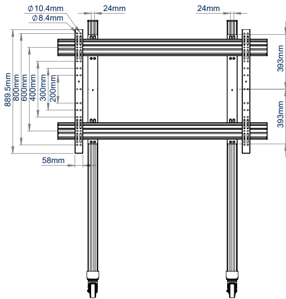
VOORAANZICHT
