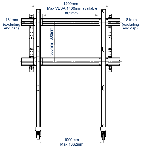
ACHTERKANT
