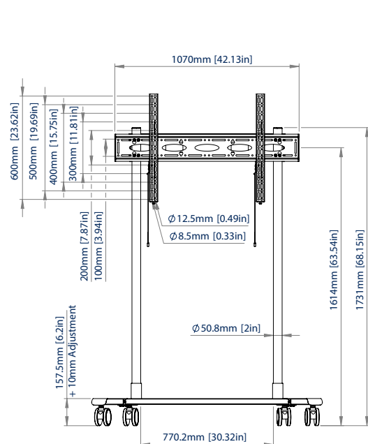
VOORAANZICHT MET CASTORS
