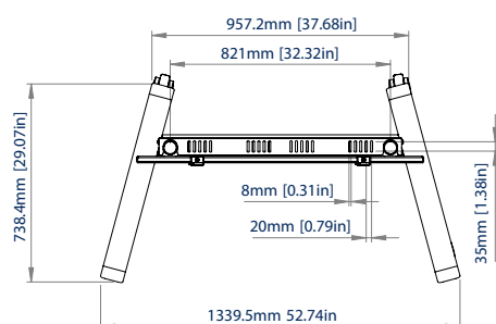
BOVENAANZICHT
