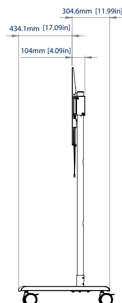
ZIJAANZICHT MET CASTORS
