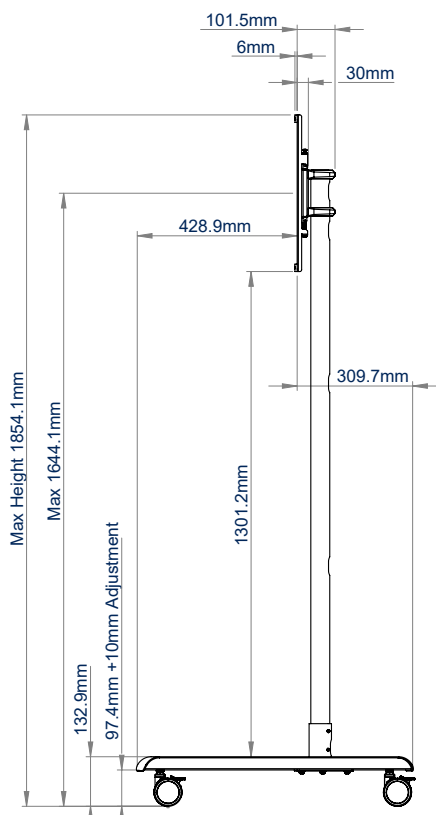
ZIJAANZICHT MET ZWENKWIELEN
