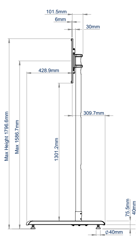
ZIJAANZICHT MET STELVOETEN
