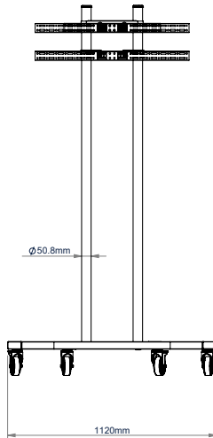
VOORAANZICHT MET CASTORS
