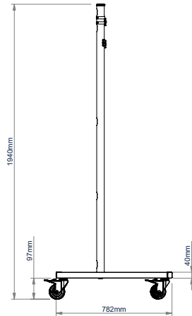
ZIJAANZICHT MET CASTORS
