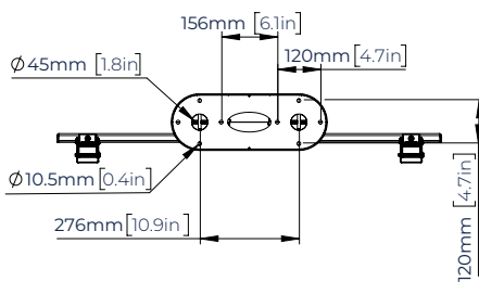
BOVENAANZICHT
