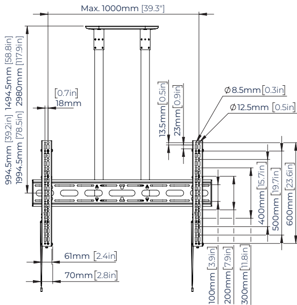
VOORAANZICHT
