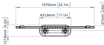
PLAFONDPLAAT – ONDERAANZICHT
