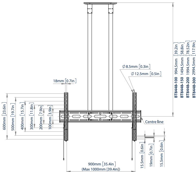
VOORAANZICHT
