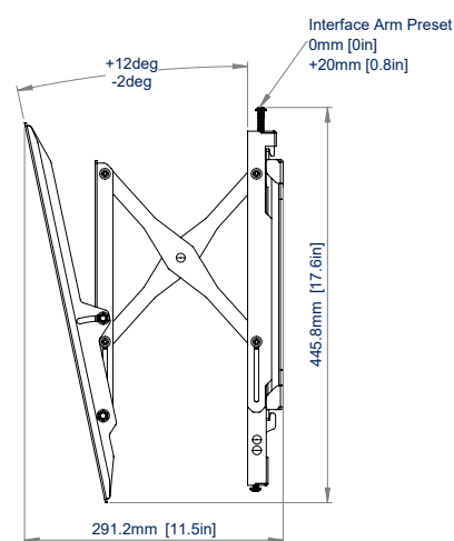
ZIJAANZICHT UITGEBREID
