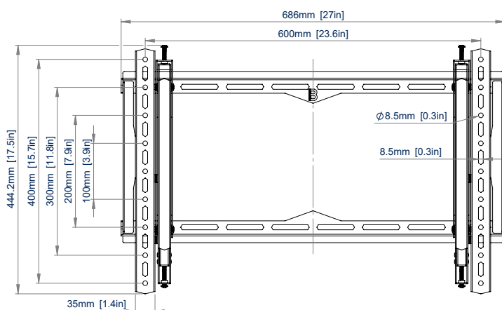
VOORAANZICHT
