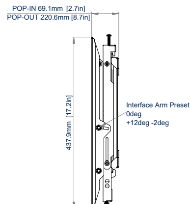
ZIJAANZICHT INGETROKKEN
