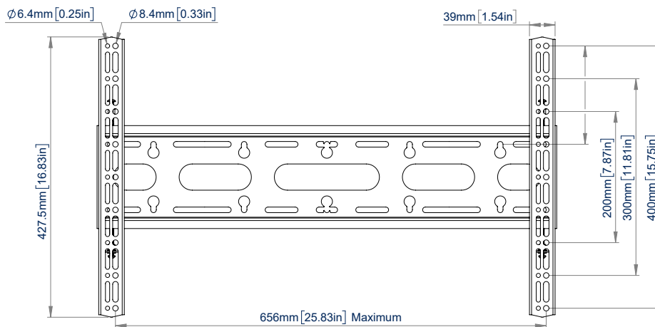
VOORAANZICHT
