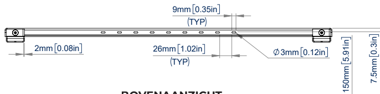
BOVENAANZICHT
