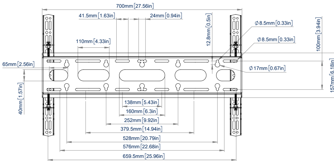
ACHTERKANT
